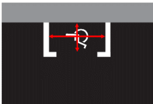
Obrázek 25 - Měření rozměrů a sklonů u podélného vyhrazeného parkovacího stání
